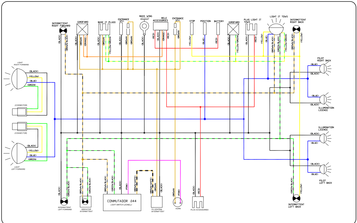
Esquema eléctrico Leonelli para manuales de instrucciones vehículo Electrical scheme Leonelli for vehicle handbook
